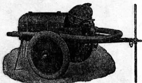
Lahka, dvokolna motorna brizgalnica z 16/18 HP motorjem, dobava vode 800 l v min., pritisk do 16 atm.
