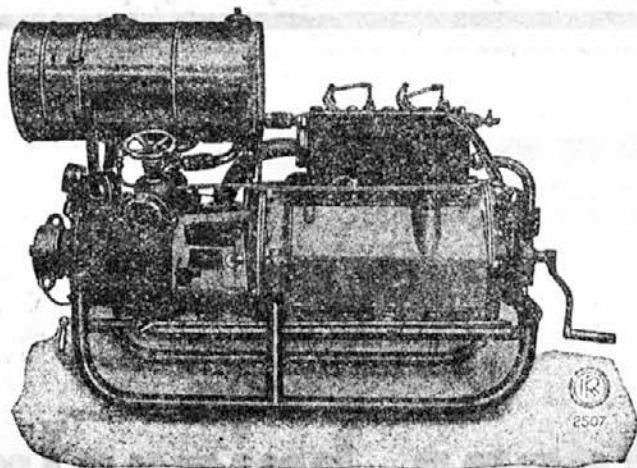
Dvocilindrska motorna brizgalnica, model 1929, 18/20 HP., pritisk do 16 atm. Hladilnik novega sistema, ogrevanje črpalke s toplo čisto vodo.
