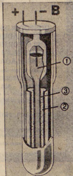
V jedru Fordovega akumulatorja je tekoči natrij (1), okrog katerega je keramični valj (2), le-ta pa je potopljen v tekoče žveplo (3). Akumulator deluje le, če celico segrejejo do temperature 300 stopinj Celzija.
