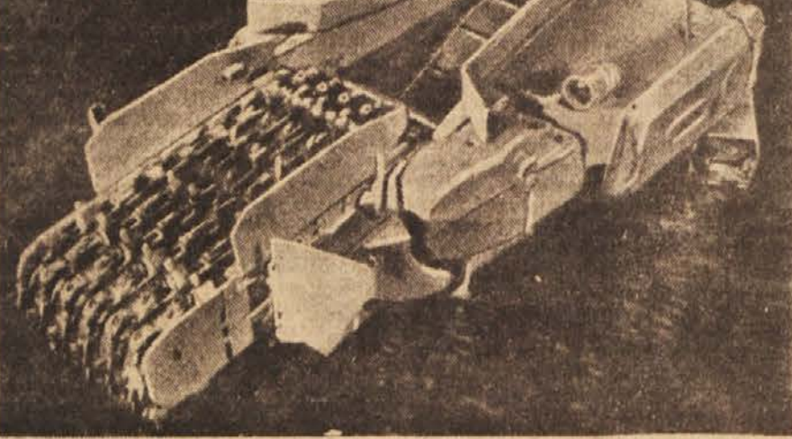
Na sliki dobro razločimo tri elemente dobivalno-nakladalnega stroja: glavo, ki se zariže v plast premoga in ga trgá, dalje srednji tekoči trak na trupu in zadnji tekoči trak na repu, ki prenašata premog na konec repa in od tam na transportni kamion. Položaj v katerem je stroj, tudi jasno kaže, kako je glavo in rep lahko obračati za 45 stopinj na levo in na desno od strojevega trupa, kar mu daje mnogo večji učinek brez premikanja z delovnega mesta.
