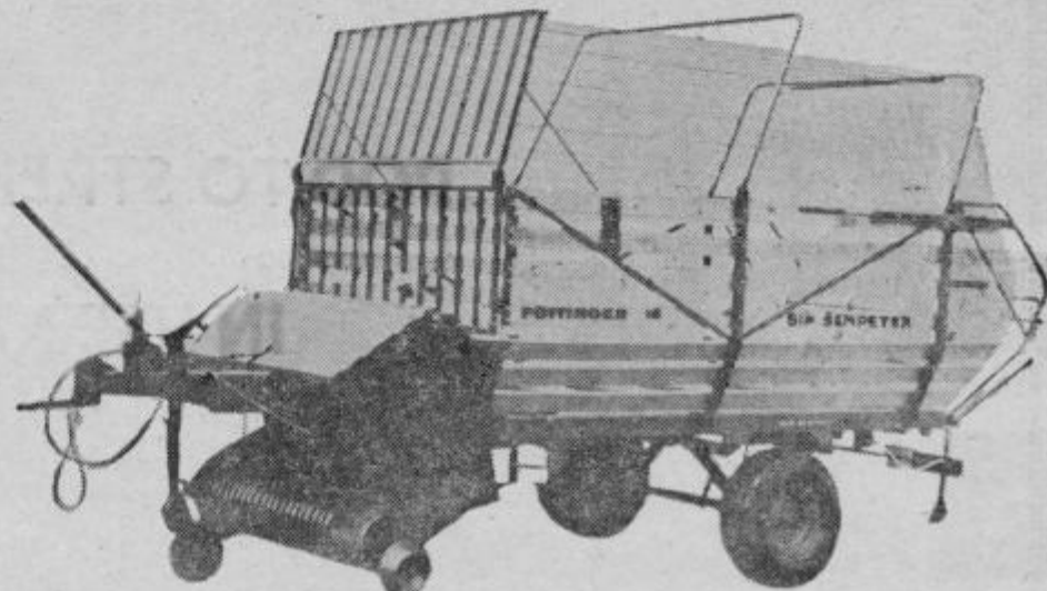
Samodejna nakladalna prikolica za nakladanje in transport zelene ali suhe krme Pirat 15 — kooperacijski izdelek Pöttinger — SIP Šempeter.
