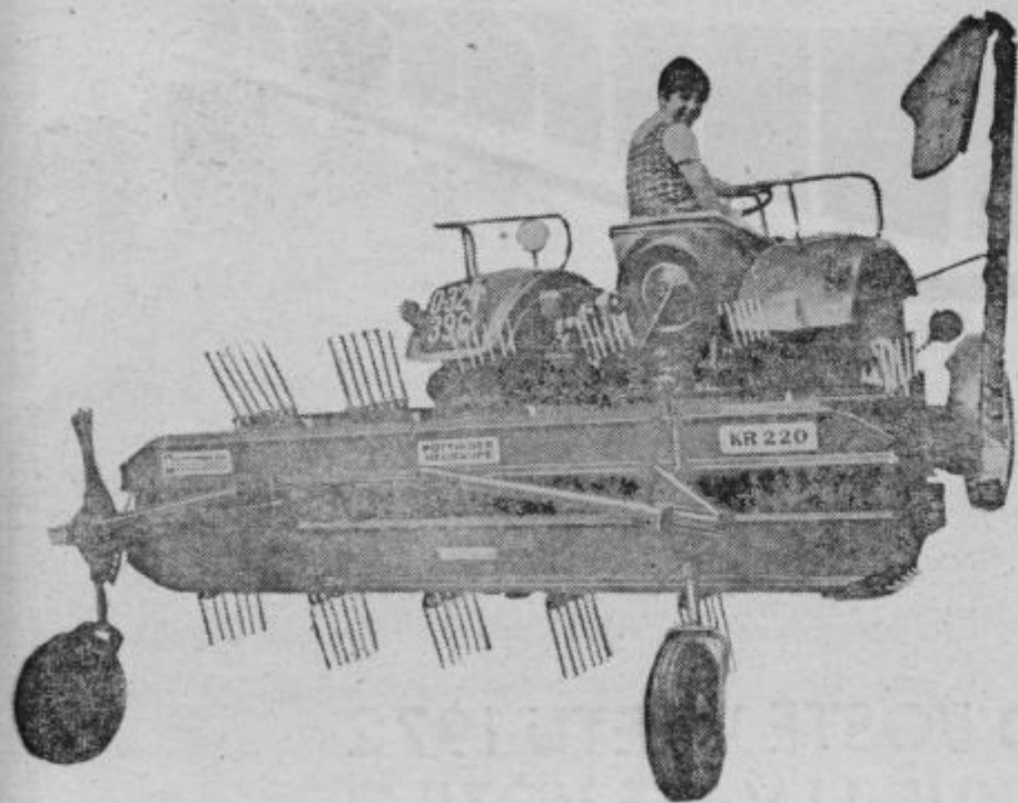
Traktorski obračalnik in zgrabljalnik za seno Favorit-220 — kooperacijski izdelek Pöttinger — SIP Šempeter
