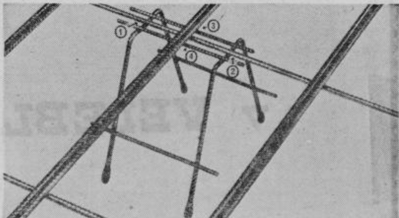
DISTANČNIKI (nosilci negativne armature za betonske plošče) DIN 1945 § 11.2 predpisuje:
