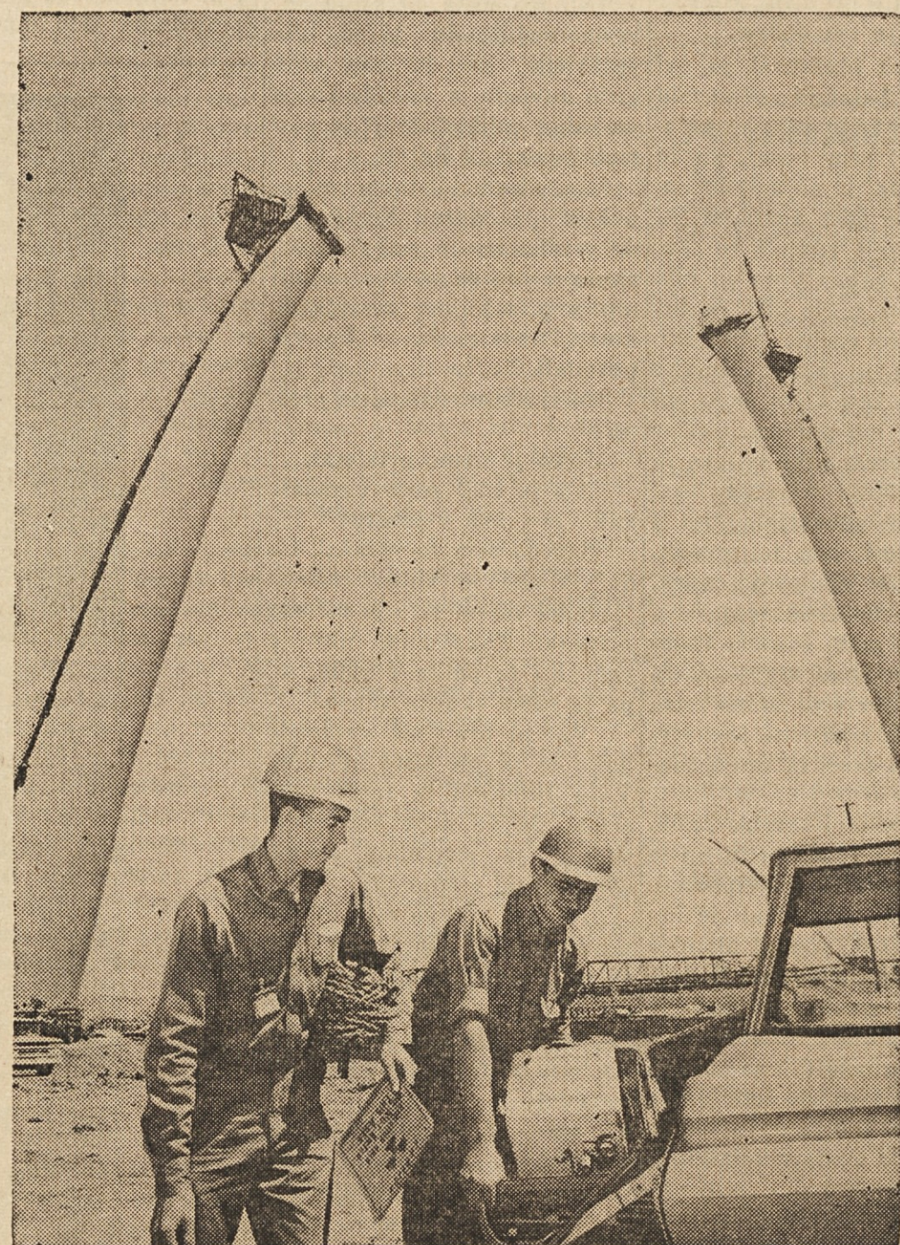
MODERNI PREGLED TRDNOSTI — Moža jemljeta iz avtomobila napravo, s katero bosta s pomočjo gama žarkov pregledala trdnost obeh stebrov "vrat" na Zahod v St. Louisu. Z navadnim očesom morebitnih poči v jeklu ni mogoče opaziti.
