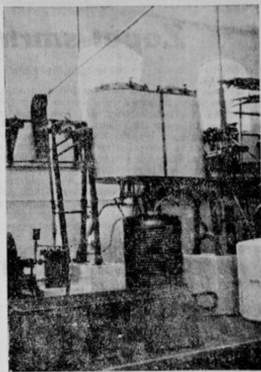
Biorizacijska aparatura: V ospredju vidimo kad, v katero se izteka mleko iz cedila. Na vrhu aparature vidimo 2 biorizacijska kotla in pod njima hladilnik z hladilnimi obroči.
