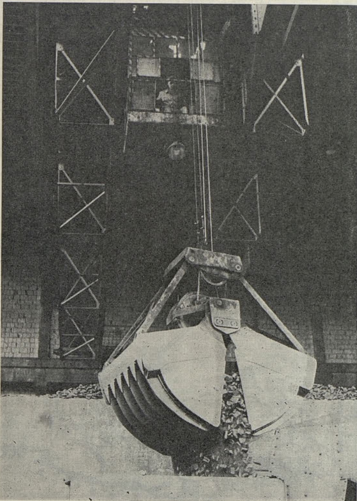
Nakladanje anodne mase
