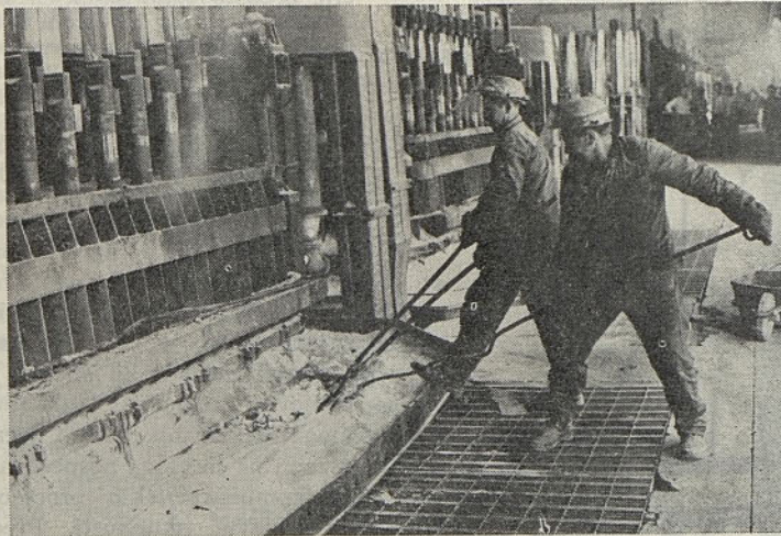
Proizvodni detajl
