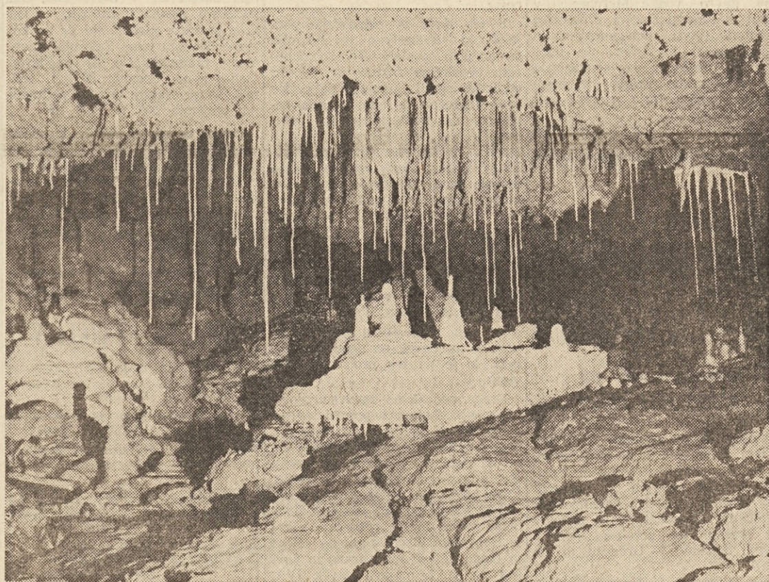
«Oltarska dvorana» v Matajurski jami
