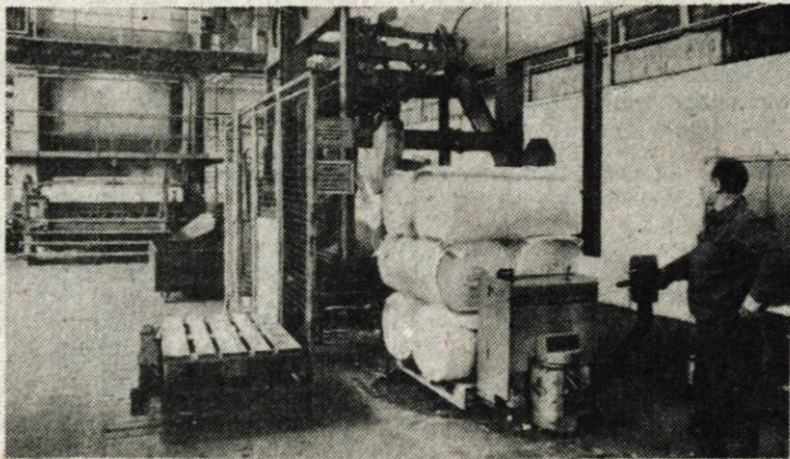
Sodobna linija za izdelovanje celuloze
