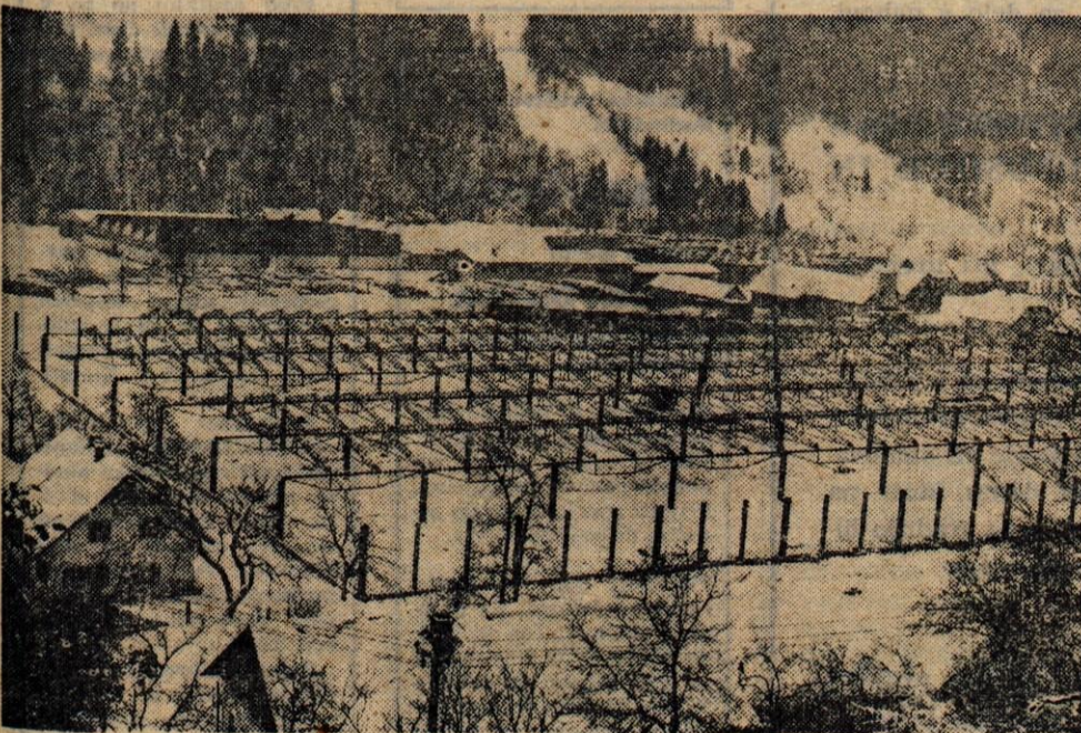
Te dni so tehniki podjetja Termika iz Ljubljane začeli s prekrivanjem nove hale tovarne Alples. Streha tega orjaškega lesnoindustrijskega obrata bo iz aluminijaste pločevine.
