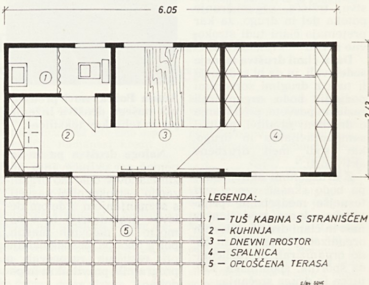
MOBILARNI BLOK—POČITNIŠKA HIŠICA
