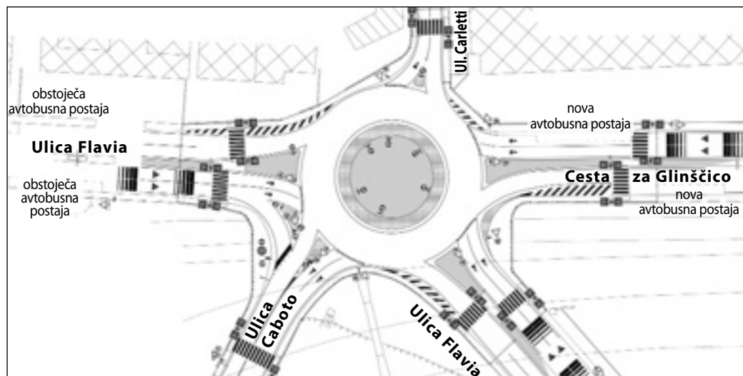
Načrt za novo krožišče
