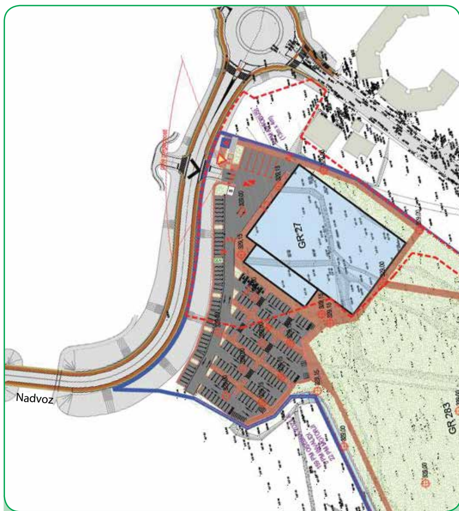
Prikaz načrtovanega nadvoza, povezovalne ceste in križišča v Sončnih dvorih
