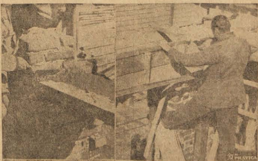
Slika levo: zidar polaga betonirano preklado; na desni: tesar pa pripravlja šele opaž za betoniranje okenske preklade po starem načinu. (O novem načinu zidanja smo poročali v četrtkovi številki.)
