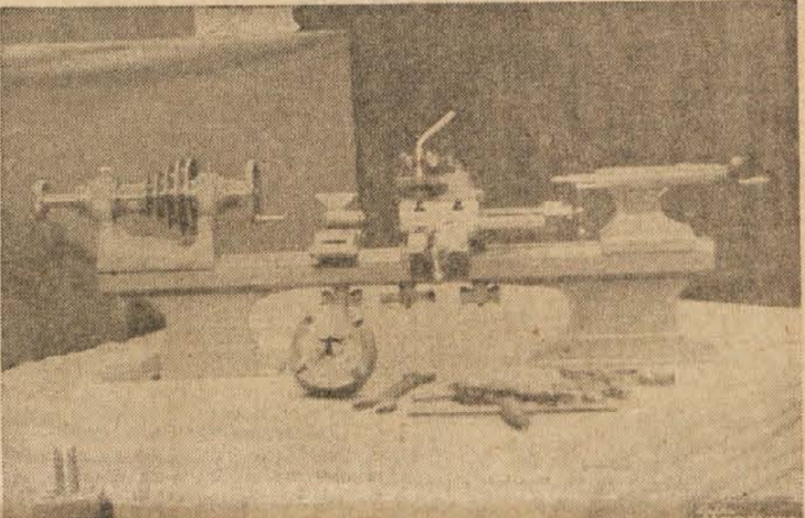
Miniaturno izdelana stružnica, delo vajencev vajeniške šole v tovarni fine mehanike »ISKRA« v Kranju. Tovrstne stružnice se uporabljajo v precizni mehaniki.
