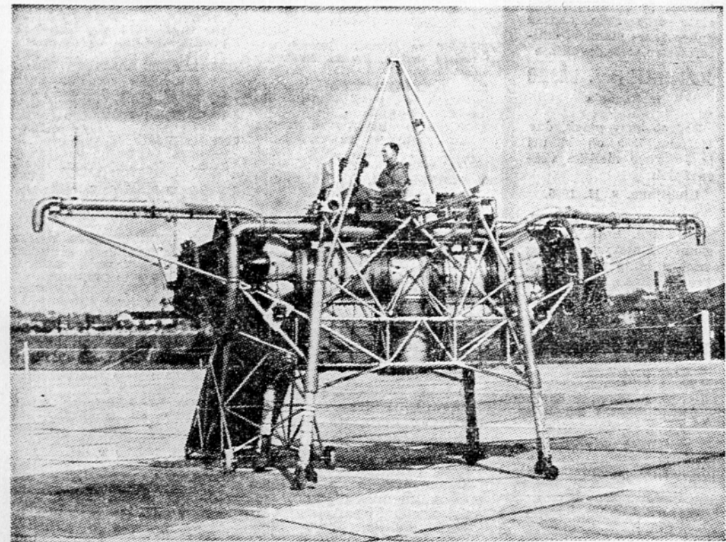
Lani v septembru je čudna naprava z imenom »leteča postelja« zbudila precejšnje zanimanje. Angleško letalstvo je pravkar objavilo tole zanimivo sliko. Naprava nima kril niti rotorjev, kot jih ima helikopter, toda kljub temu se lahko dvigne navpično z zemlje. Pogonjata jo dva reaktivna motorja »Nene«, ki sta postavljena vodoravno, drug drugemu nasproti. Reaktivni curek je iz obeh motorjev speljan pod kotom 90 stopinj proti zemlji (na sliki: čev vsredini, ki je obrnjena proti tlom), tako da deluje točno v težišču. Pilot sedi na ploščadi nad obojema motorjema in manevrirna napravo s pomočjo stisnjenega zraka, ki ga pušča skozi dolgi cevi na obeh straneh ogrodja.
