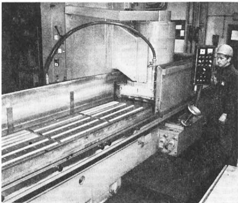
Brušenje nožev
