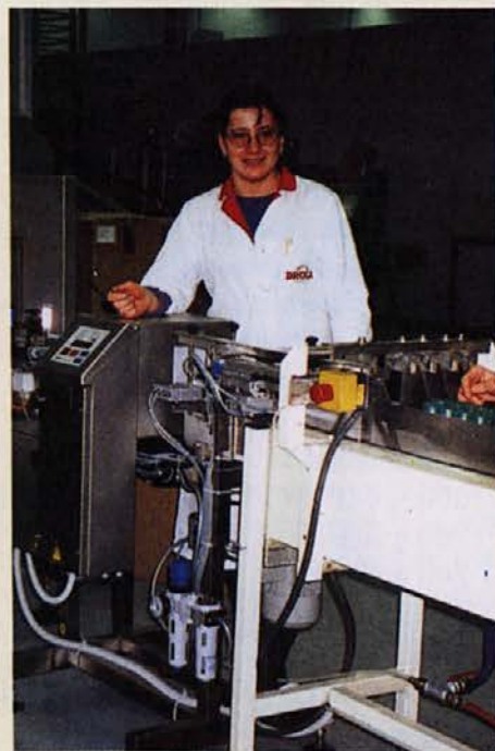
Na liniji za pakiranje začimb v stekleničkah je vgrajen detektor kovin
