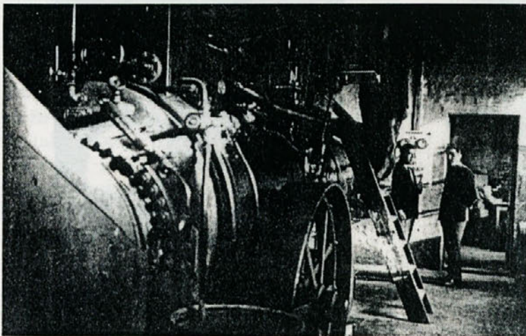
Kebetova žaga v Vipavi 1929. leta, lokomobila je imela moč 160 KS. Na sliki desno Jože Kebe, na levi Franc Kebe in v ozadju za pisalno mizo Marija Grabrijan.
