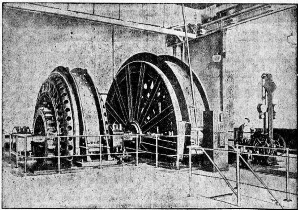
Največji dvigalni stroj na svetu imajo Nemci. Premer ogromnega kolesa meri 7,5 m. Stroj ima moč 10.000 konjskih sil. V eni uri s pomočjo tega stroja lahko dvignejo iz globine 1050 m 545 ton premoga, ali v enem dnevu, če teče stroj samo 14 ur, približno 140.000 metrskih stotov.
