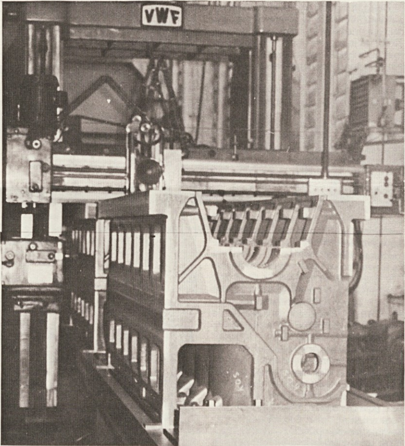
Prednostna proizvodnja so letos vsekakor dizel motorji. Skozi obdelavo je šlo letos že več kot 40 ohišij. Na fotografiji je obdelava zgornjega dela ohišja 6-cilindrskega dizel motorja za Uljanik iz Pule, ki je naročil 4 motorje te vrste (Foto: E. L.)
