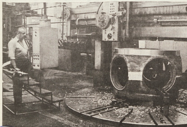
Obdelava glave Kaplanovega gonilnika za HE Mostar na kopirni pokončni stružnici. Teža glave je okoli 5 t. V HE Mostar bodo instalirani trije takšni agregati s skupno močjo 80 MW. (Foto: E. L.)
