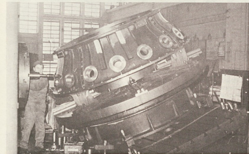
Obdelava ležajnih izvrtin na zunanjem vodilniku za cevno turbino Fužine pri Ljubljani. HE Fužine spada po moči v srednji razred. Instaliran bo samo en agregat in bo pri padcu 6 m imel moč 900 KW (Foto: E. L.)
