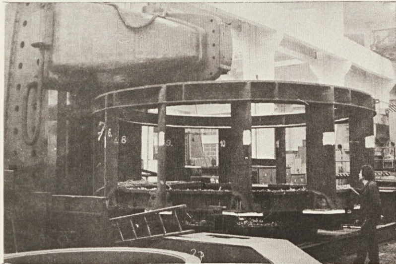
Struženje predvodilnika za drugo turbino HE Mostar. Teža predvodilnika je 20 t, premer pa skoraj 7 m. HE Mostar je po svojih značilnostih zelo podobna HE Mavčiče, le da bo imela en agregat več in bo zato tudi za eno tretjino močnejša. Vsa dela za HE Mostar potekajo v roku.
