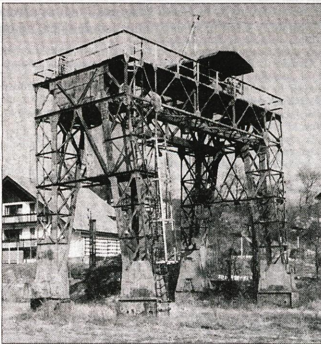
Portalni žerjav z začetka tega stoletja naj bi stal ob vhodu v muzejsko kulturni kompleks na Stari Savi. Foto: Muzej Jesenice
