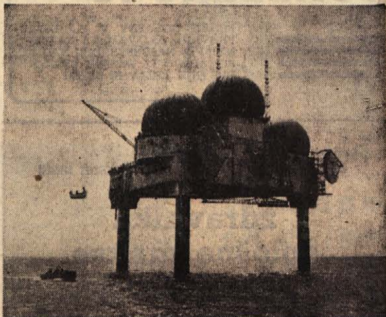
Okoli 120 km severovzhodno od ameriške atlantske obale je »r-darski otok«, na katerem ima ameriško vojno letalstvo opazovalnico. Ogrodje umetnega otoka ima obliko trikotnika s 60 m dolgimi stranicami
