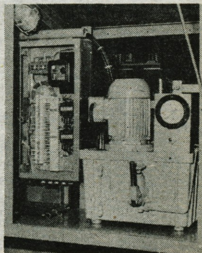
V elektrodalavnici so izdelali omarico za avtomatsko delovanje čistilnega stroja in upravljanje zapornice za izpust vode.
