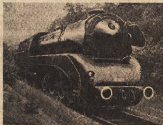
V Nemčiji preizkušajo novo parno lokomotivo. Ima tri cilindre, ki zmogajo 2500 KM. Lokomotiva doseže hitrost 145 km in se sama oskrbuje z elektriko. — Na ozemlju Zahodne Nemčije obratuje zdaj še kakih 7000 parnih lokomotiv
