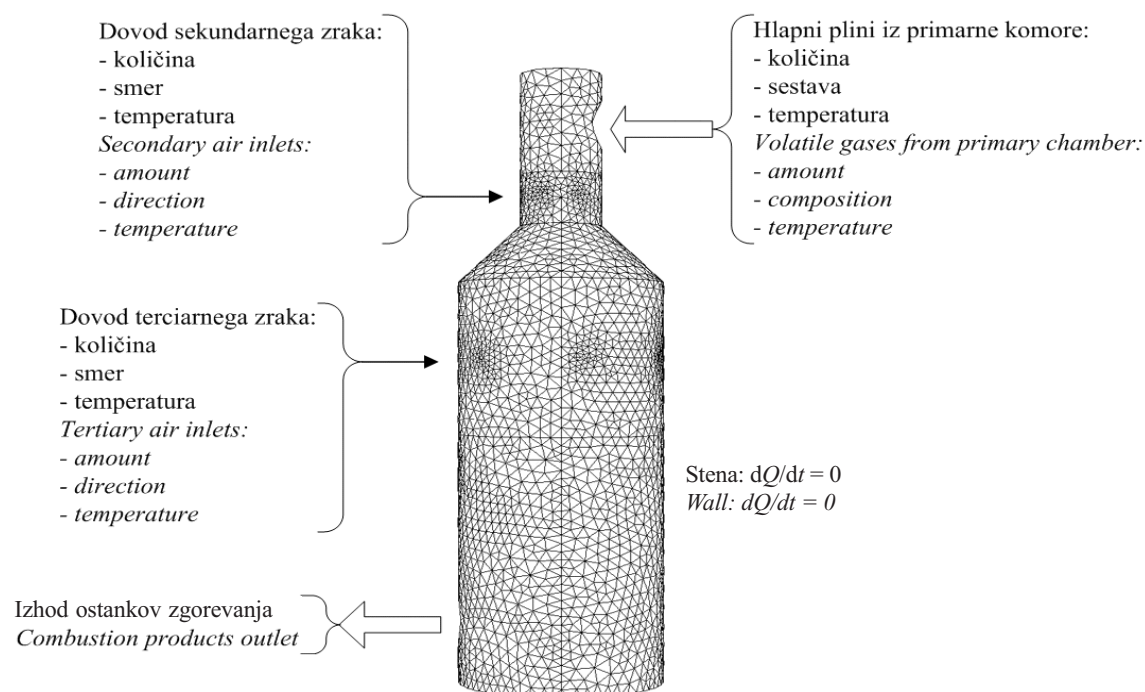
Sl. 2. Robni pogoji in zamrežitev termoreaktorja
