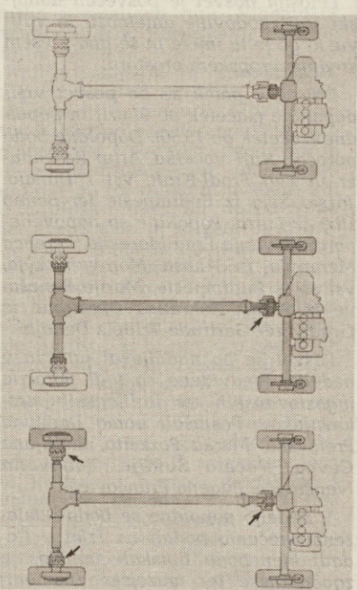
Schema prehoda od pogona 4x2 k pogonu 4x4
