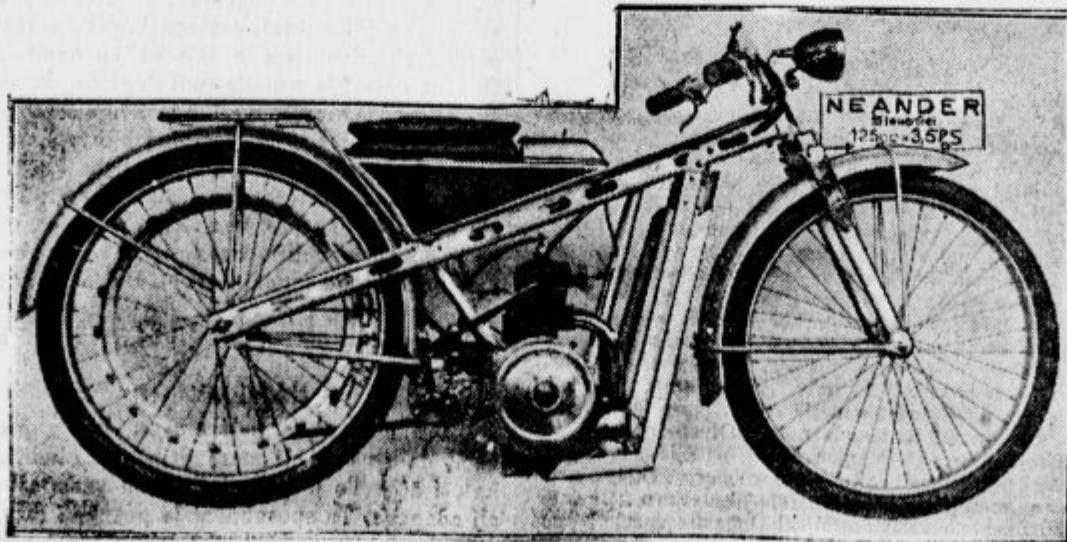
Zanimiva nova konstrukcija v izdelovanju motornih koles. Okvir obstoji iz lahkih železnih nosilcev.
