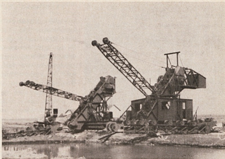
Gradnja prekopa Donava - Tisa - Donava s pomočjo modernih strojev
