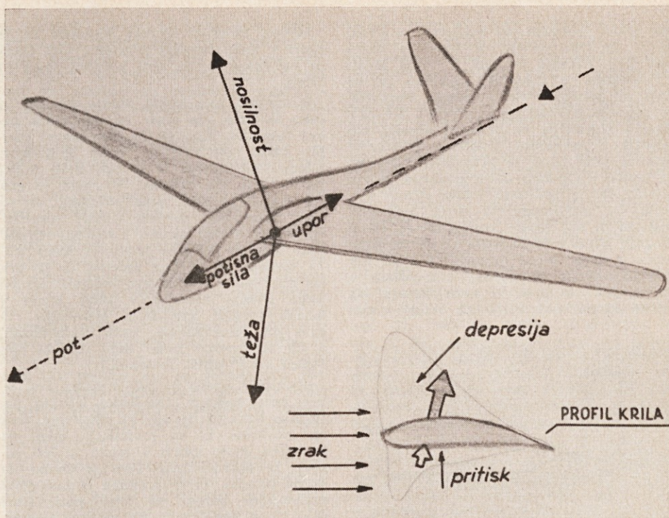
Komponente sil, ki delujejo na let jadralnega letala
