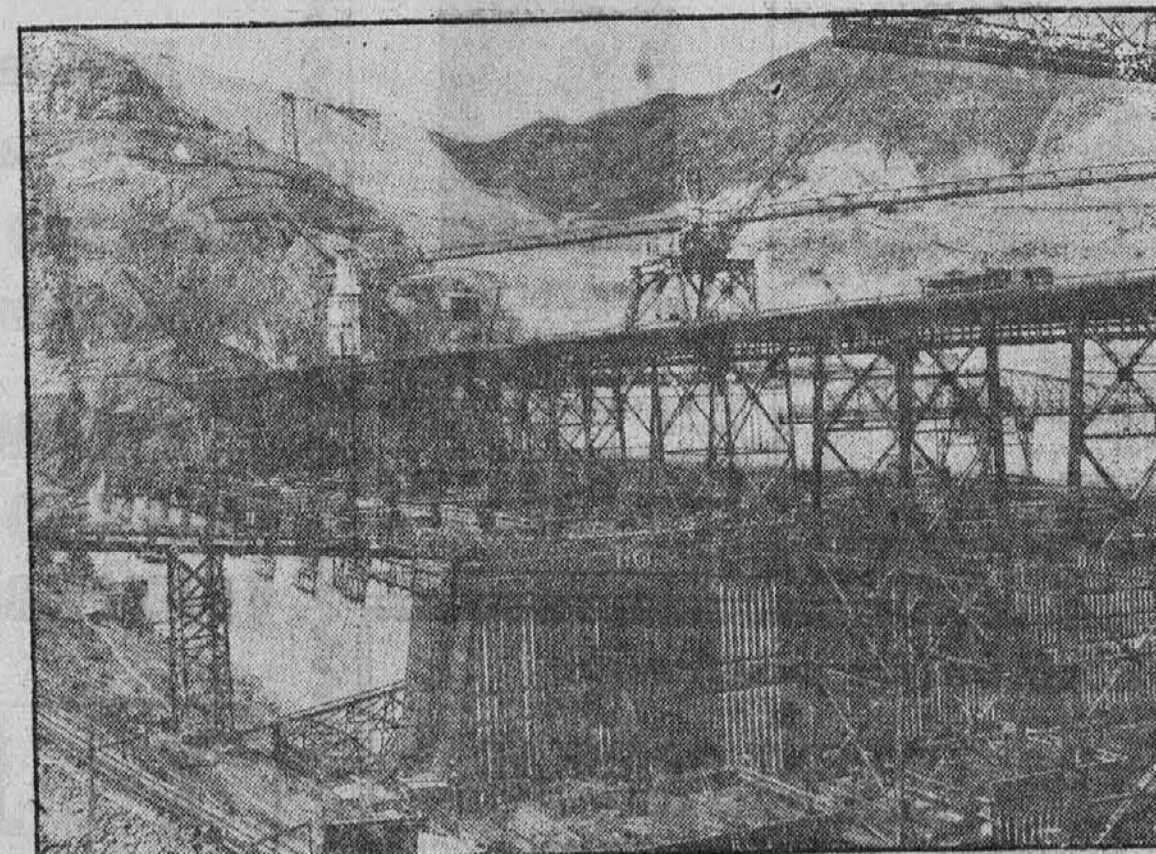
V državi Washington so začeli Columbia reko, kjer zidajo velik Coulee jez. Jez bo stal $63,000,000. S pomočjo te vode bodo umetno namakali 2,000,000 akrov zemlje, ki je zdaj puščava in jo bodo spremenili v rodovitno zemljo. Jez bo 430 čevljev visok in 4,290 čevljev dolg. Voda se bo dvignila 151 milj daleč v reko.
