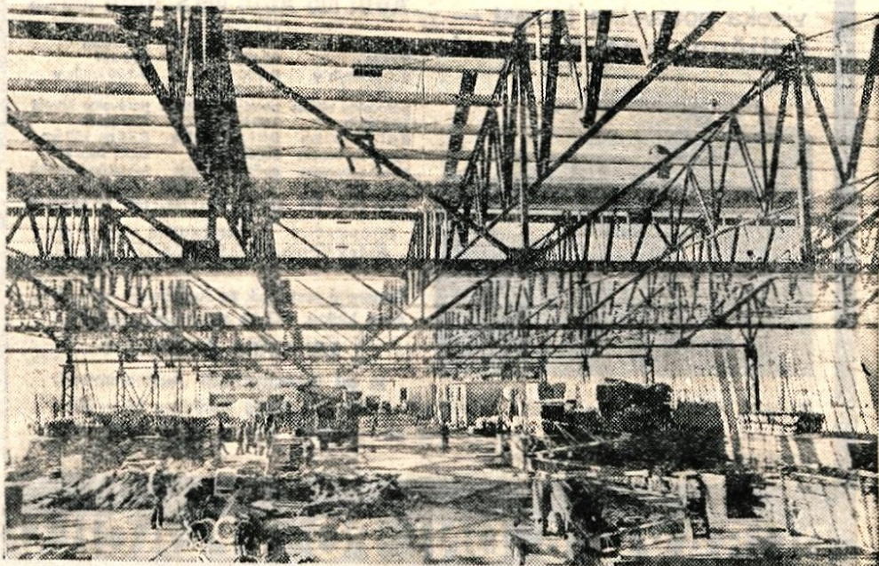
Ob cesti Škofja Loka—Trata gradi podjetje Jelovica okrog 6000 kvadratnih metrov veliko lo-po za vskladiščenje žaganega lesa. V lopi bodo uredili tudi sušilnice, brusilnice in kompresorsko postajo. Konstrukcijo, ki je na sliki lepo vidna, postavlja podjetje Metalna iz Maribora, gradbena dela izvaja Tehnik Škofja Loka, notranja opravila, napeljavo in podobno pa so prevzela številna druga manjša slovenska podjetja (-ig) — Foto: F. Perdan
