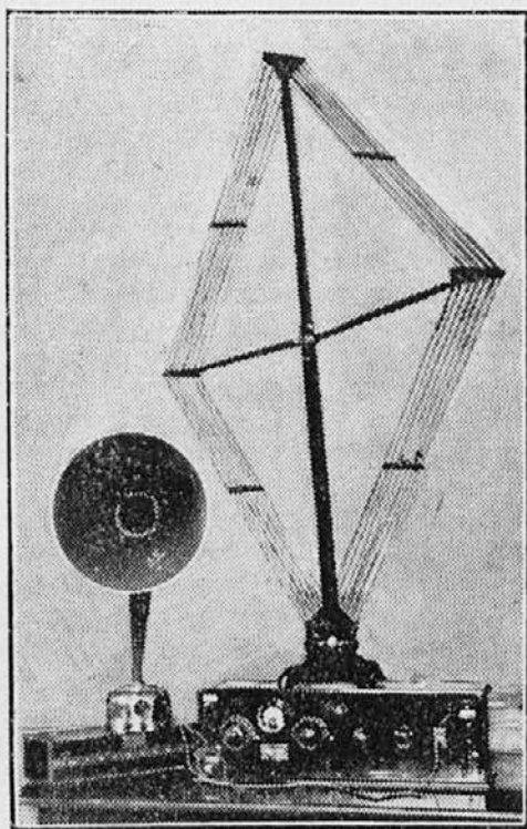
Radiopriprava z okvirno anteno in zvočnikom.
