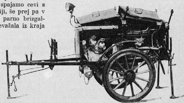
Dvokolna priklopna motorna brizgalnica.
