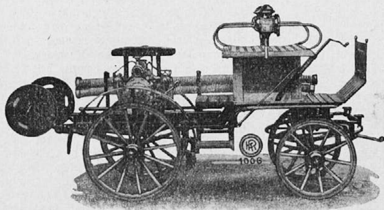
Četverokolna motorna brizgalnica za konjsko vprego (Rosenbauer).
