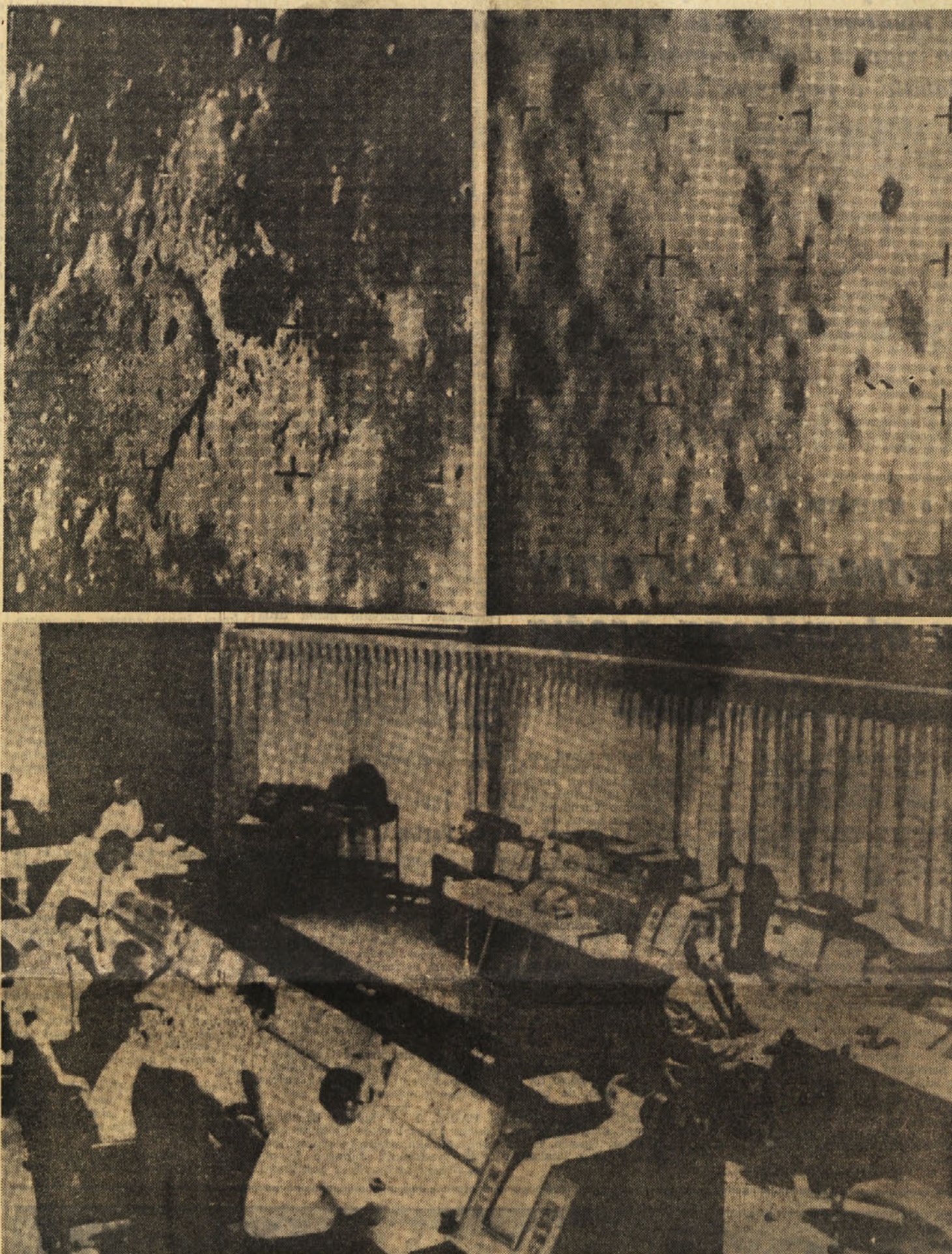
Zgoraj: Lunina površina, kakor jo je slikal »Ranger VII« ko je bil oddaljen od nje približno 300 metrov.
