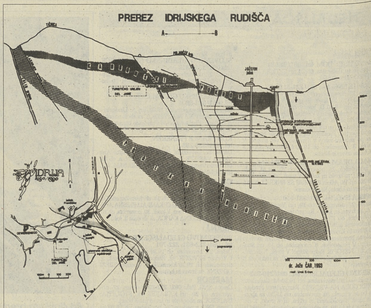
Shema zapiranja rudnika živega srebra
