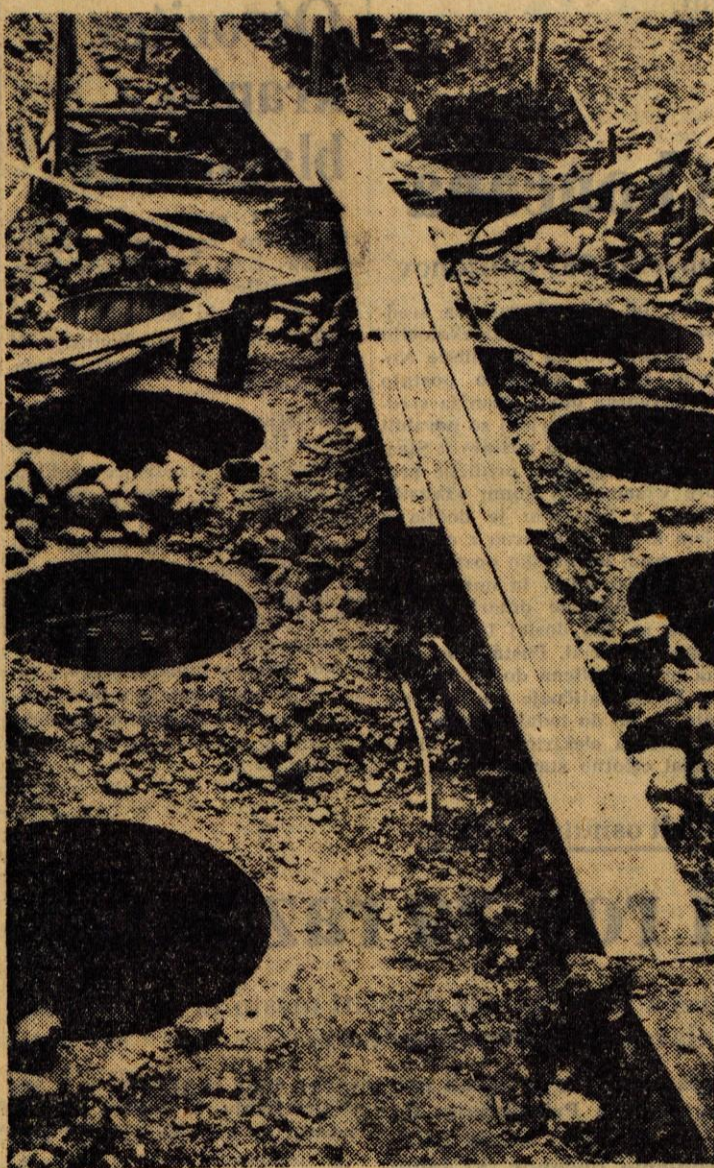
Pogled na gradnjo tako imenovanih »vodnjakov« — temeljev za novo tržiško stolpnico
