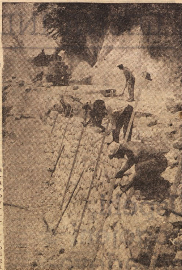
Vzporedno z rekonstrukcijo kamnoloma so morali kresniški apnarji zgraditi tudi novo cesto. Pri gradnji opornil zidov za novo cesto, ki peljejo v kamnolom
