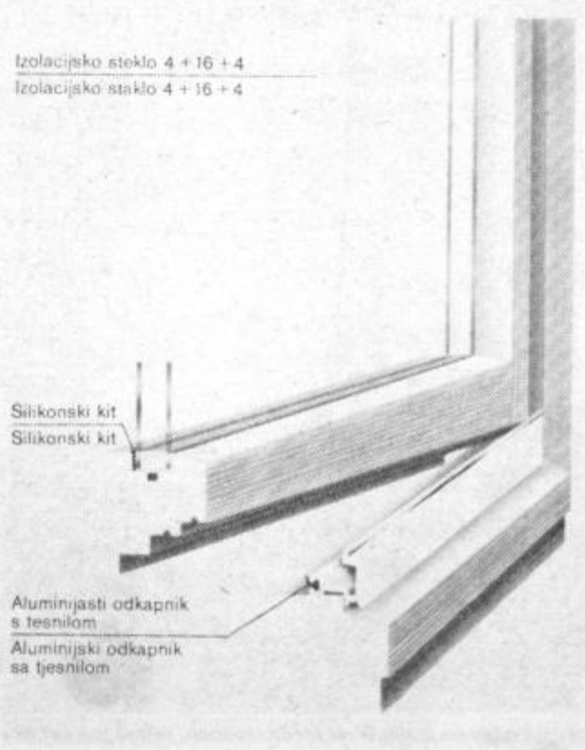
Prerez termo okna.
