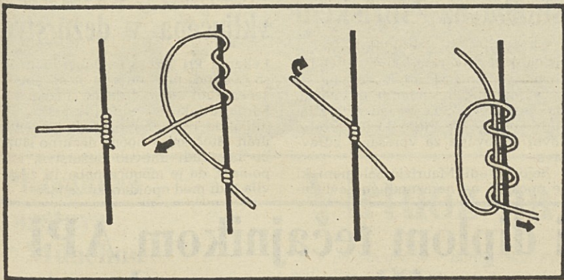
S tem vozlom bomo na glavno najlonsko vrvico privezali tanjše vrvice s trnki.
