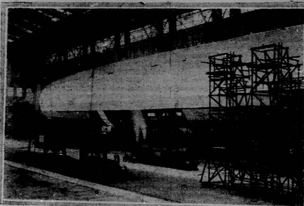
V Lakehurst, N. J., so dogradili velikanski mornariški balon ZR-1. Dne 1. septembra se bo prvič dvignil v zrak. Čitatelji si lahko predstavljajo, kako je zrakoplov velik, če primerjajo z njim železniško lokom otivo, ki stoji poleg njega.
