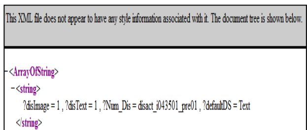
Figure23:Display_check result
