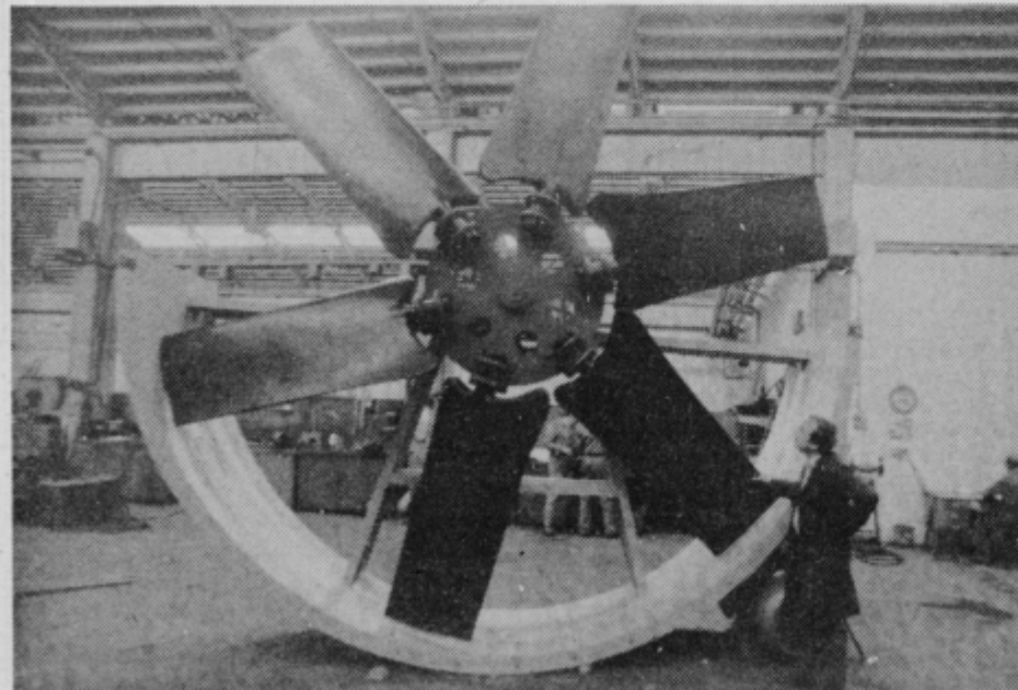
Aksialni ventilator, premera 4,5 metra, za hlajenje v hladilnem sistemu tovarne sladkornja Tuzla.
