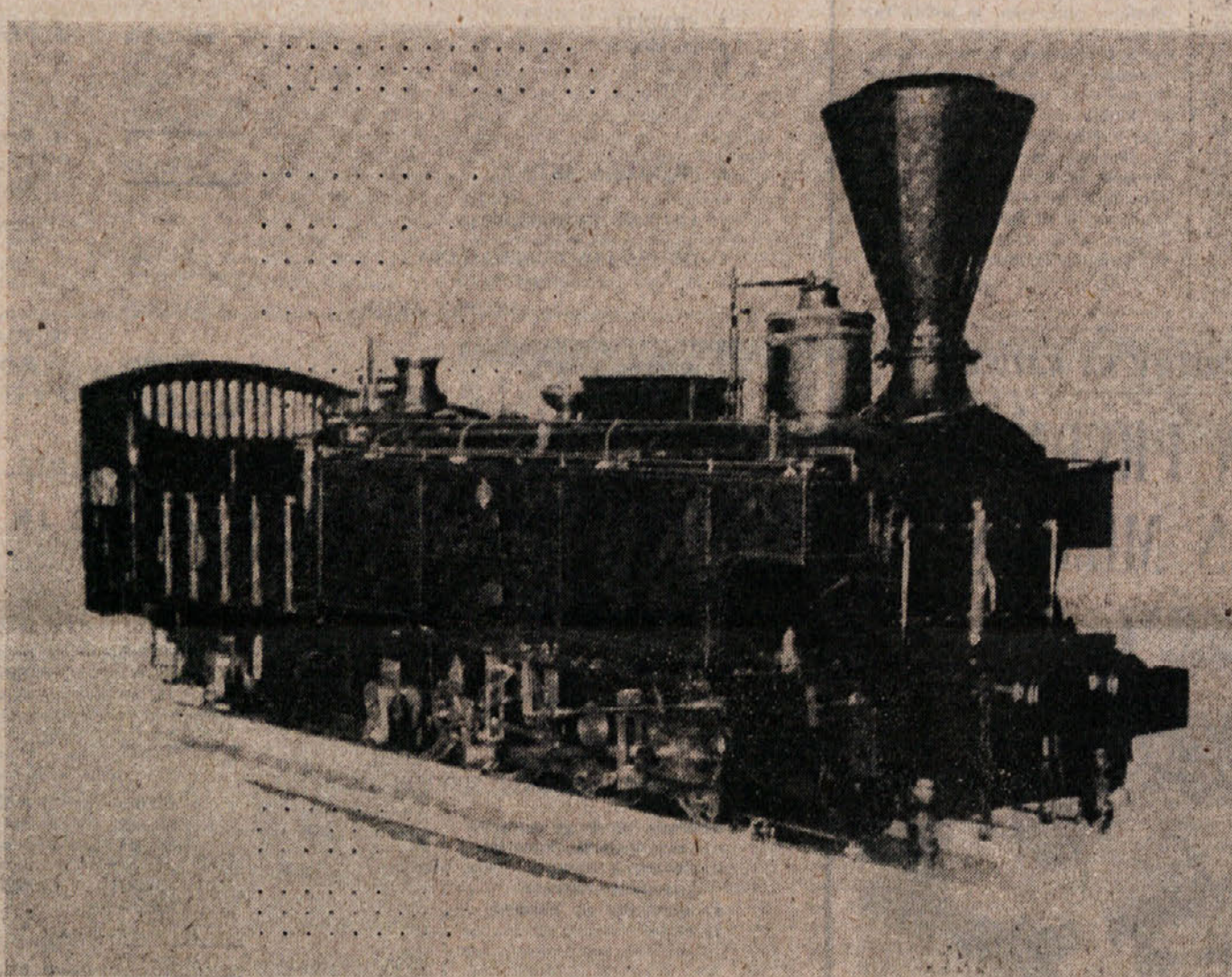
Takšne so bile gorske lokomotive »Engertha«, ki so jih po prvi svetovni vojni uporabljali le še kot premikalce. Vlekle so vagona po klancih našega Krasa.
