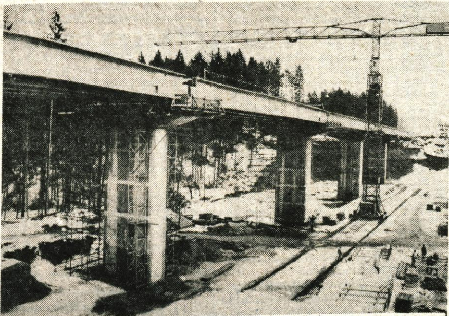
Viadukt Rupovščica na gorenjski avtocesti — Med največje projekte v Sloveniji, ki morajo biti letos gotovi, sodi prav gotovo avtocesta Nako-Ljubljana. Ena od pomembnih nalog v dinamiki del pri gradnji avtoceste je bila tudi tako imenovana težka montaža na nosilcih viadukta Rupovščica. Po programu bi morala biti ta dela končana v začetku decembra. Zaradi manjših zakasnitev na celotnem odseku trase avtoceste pa so bila ta dela končana približno teden dni pred koncem minulega leta. Izvajalcem torej uspeva dokaj uspešno loviti dinamiko gradnje. — A. Ž. Foto F. Perdan
