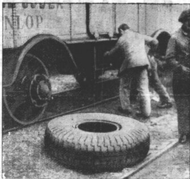
PO CESTI IN TRACNICAH. — Neka francoska prevozna tvrdka je dala napraviti novo vrsto transportnega voza. Na cesti se pomika vozilo s kolesi iz gume, na postaji pa ta kolesa zamenjajo z železnimi in voz drči po tiru kakor navaden vagon
