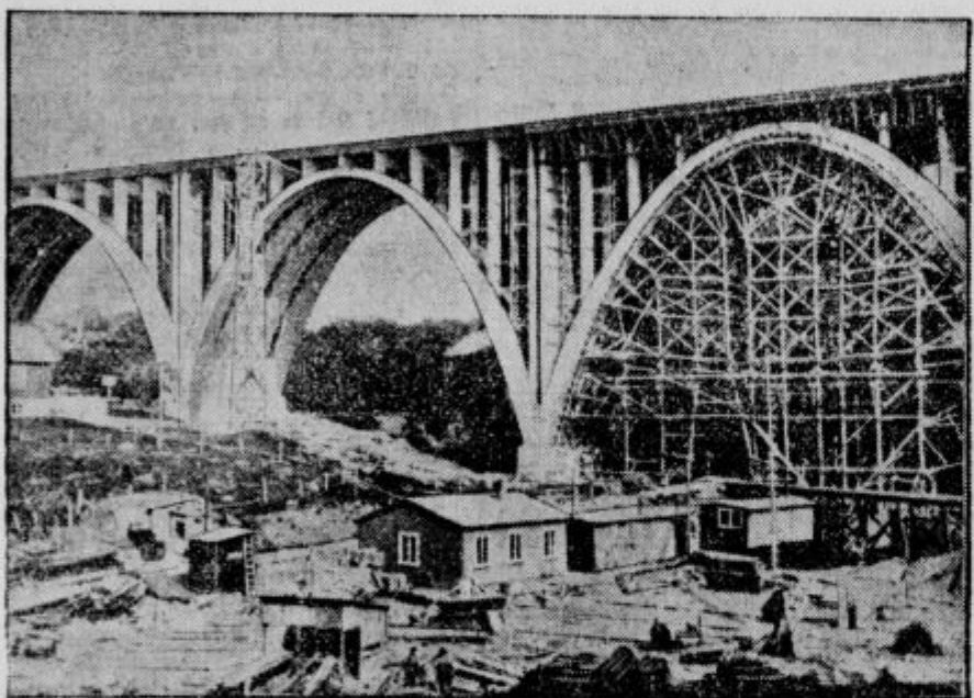
1200 m dolgi most čez Mali Belt, ki bo vezal danski provinci Jütland in Fünen. Po njem bo položen žel. tir, zraven pa bo tekla cesta za avtomobile in pešce.
