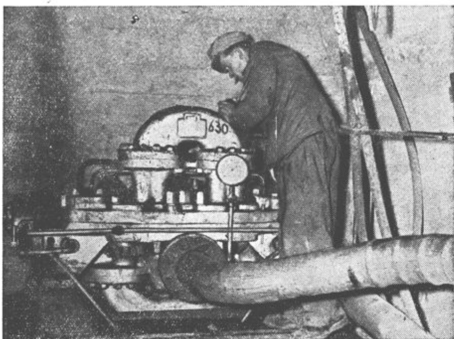
Vodna črpalka pod novim jaškom
