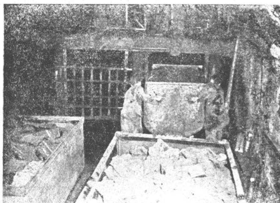
Narivanje polnih vozičkov v kletke pod starim jaškom
