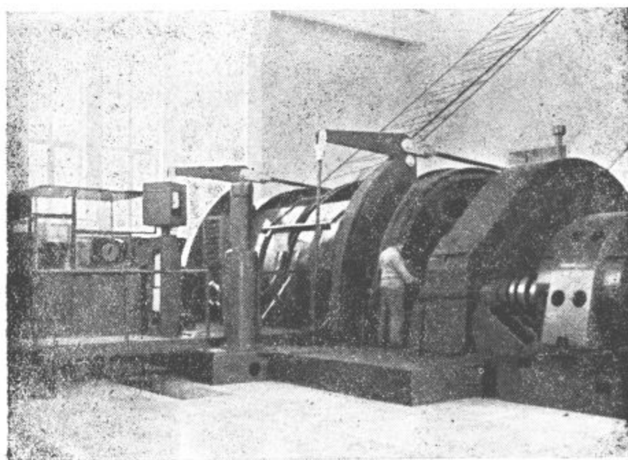
Najmodernejši izvozni stroj pri novem jašku
