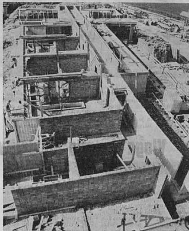
Pogled na gradbišče telovadnice in vrtca
