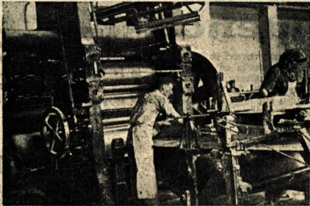
Delo pri trivlačnem kalandru
