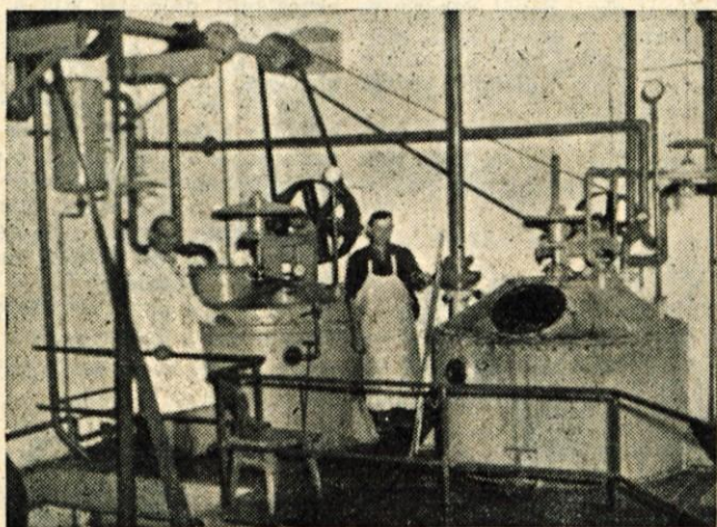
Pogled na rafinerijo »Oljarice« v Britofu
