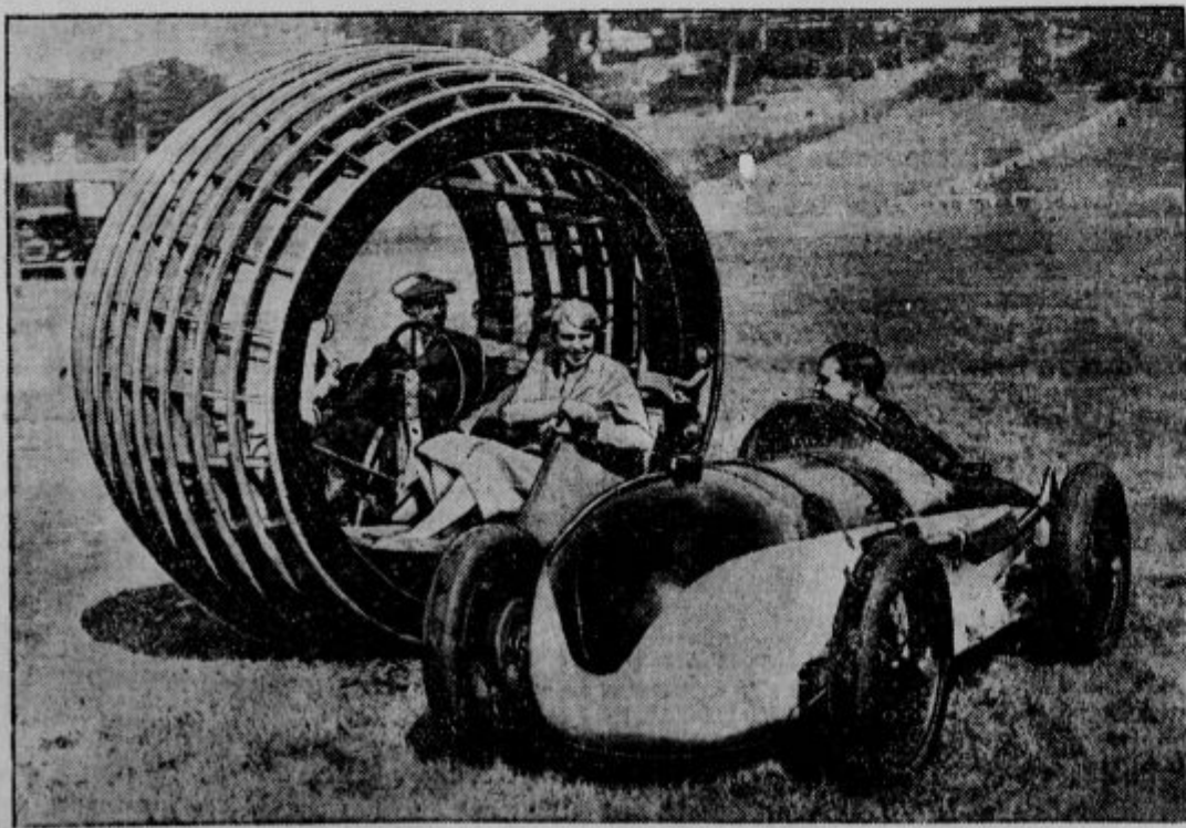
Tekma posebne vrste. »Dynamaspha«, posebne vrste vozilo, ki se pomiče samo na enem kolesu, zruven njega tipičen dirkalni avto. Sicer je avto zmagal, vendar je dosegla »dynamaspha« 50 km na uro. Pogon novega vozila vrši motor na petrolej. Šoferski sedež v notranjosti kolesa se radi lastne teže ne vrti s kolesom, marveč ostane v isti legi.
