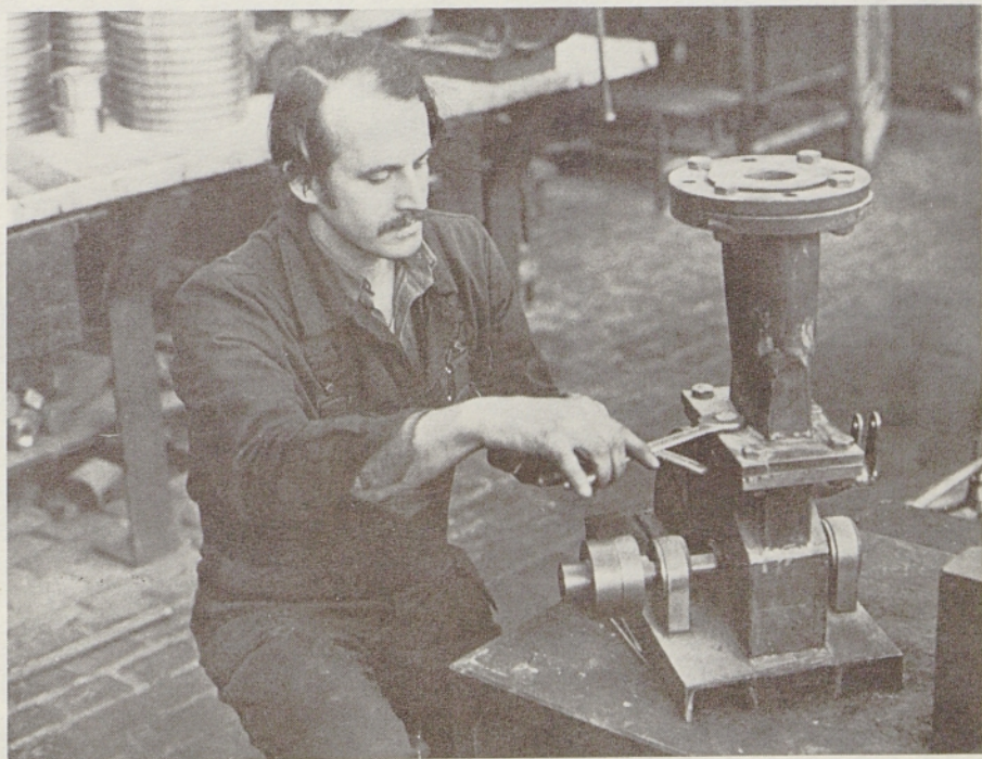
Ljubljanski Litostroj namerava začeti izdelovati manjše turbine različnih moči, ki bodo lahko v uporabi v številnih majhnih električnih centralah. – Litostroj je sicer znan proizvajalec turbin, ki so bile doslej montirane že v številnih deželah po svetu. Na sliki: Jernej Mlinar, monter turbin v Litostroju, ob prototipu male Bankijeve turbine (foto: Janez Zrnec)
