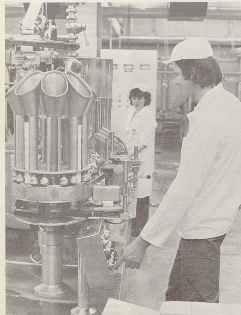
Nova mlekarna v Vipavi – stroj za polnjenje jogurta (foto: Janez Zrnc)
