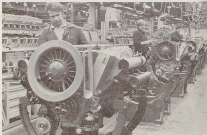
Montažna linija motorjev v TAM
