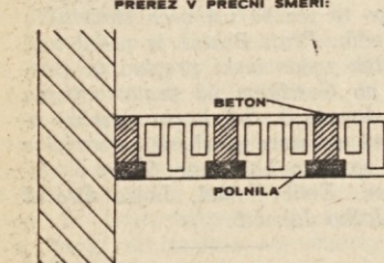
Prerez v prečni smeri:
