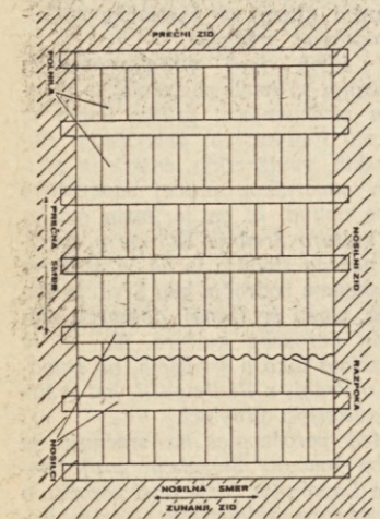
Prerez v nosilni smeri:
